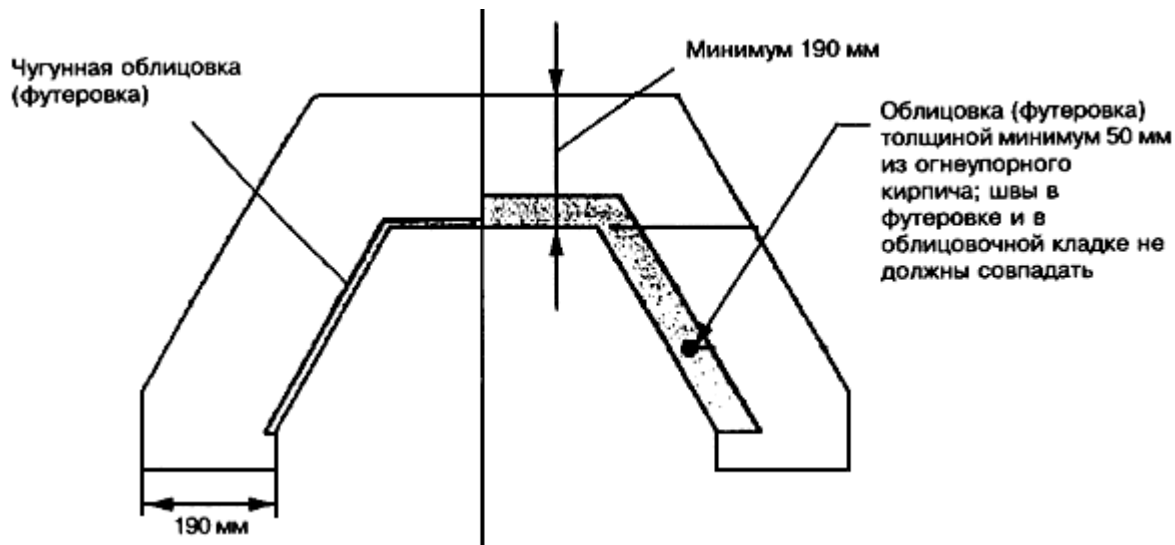
Рисунок 7.5 - Футеровка камина
