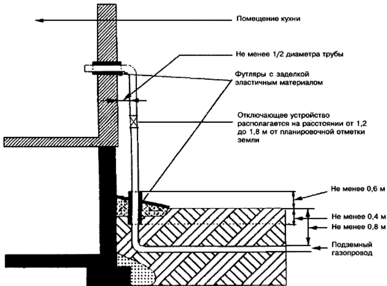
Рисунок 9.1 - Газовый ввод
