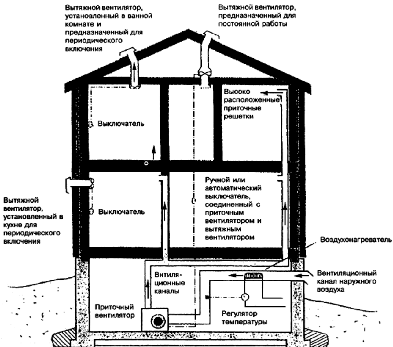
Рисунок 7.2 - Система воздушного отопления с принудительной циркуляцией воздуха, совмещенная с системой механической вентиляции, не присоединенная к системе теплоснабжения
