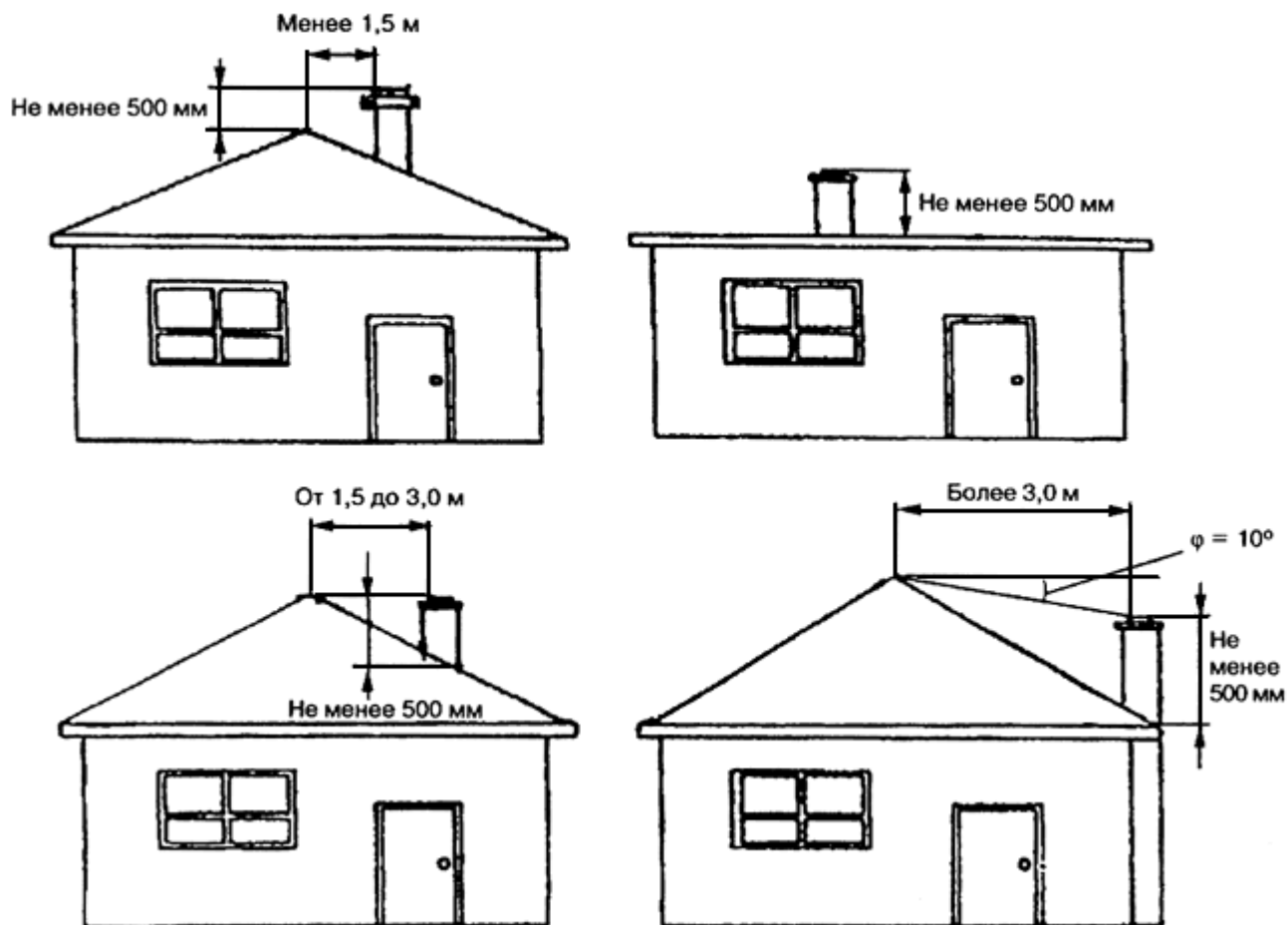
Рисунок 7.9 - Минимальная высота дымовой трубы
